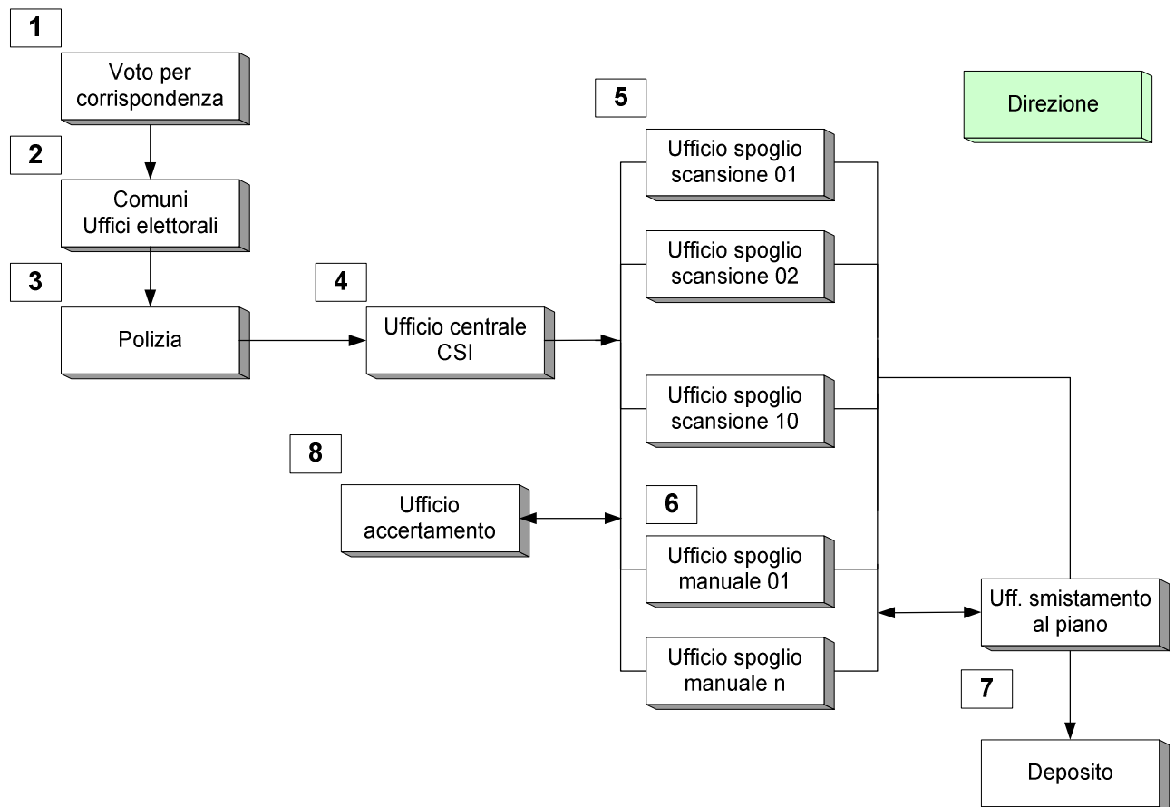
Figura 1: Flusso delle operazioni di spoglio
