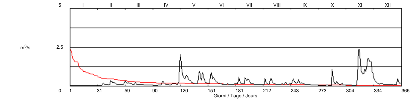
Andamento delle medie giornaliera Ganglinie der Tagesmittel Hydrogramme des moyennes journalières Curva di durata delle medie giornaliera Dauerlinie der Tagesmittel Courbe des valeurs des moyennes journalières
