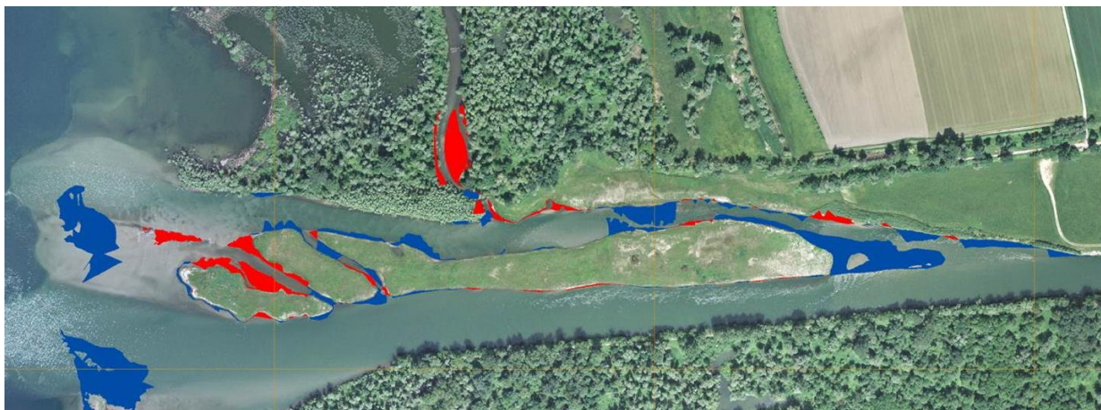
Visualizzazione delle aree di erosione (blu) e deposito (rosse) al di sopra della quota 193.5 m slm, confrontando la situazioni 2010 – 2015.
