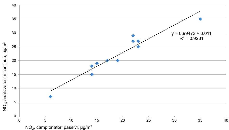
Figura 4: Confronto delle concentrazioni di NO 2 rilevate con i campionatori passivi e gli analizzatori in continuo per l'anno 2021. La linea rappresenta la curva di regressione lineare
