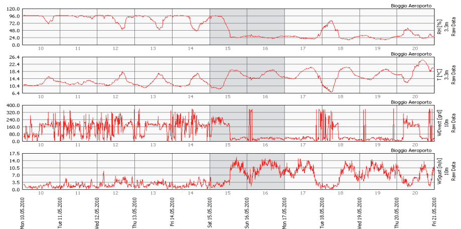
Figura 34: Dati meteorologici della stazione di Bioggio, dall'alto in basso: umidità relativa (RH), temperatura (T), direzione (WDvect) e velocità (WSgust) del vento.
