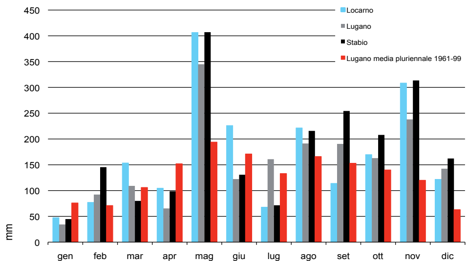
Figura 6a: Somma delle precipitazioni mensili
