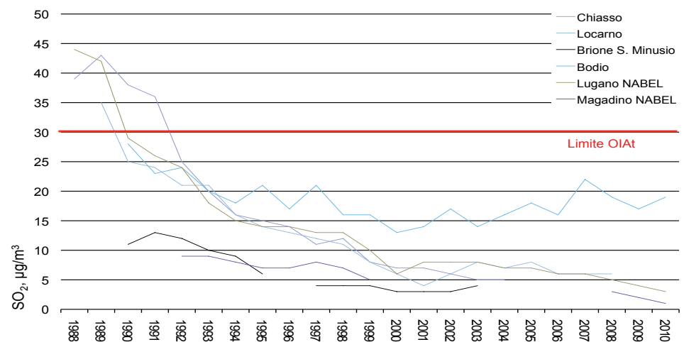
Figura 17: Evoluzione delle medie annue di diossido di zolfo in Ticino, 1988-2010
