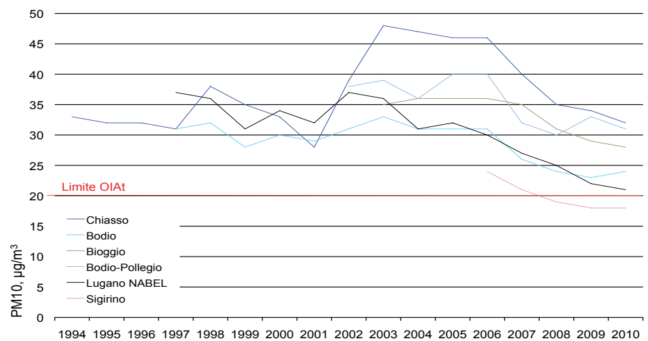
Figura 24: Evoluzione delle medie annue delle polveri sottili, PM10, in Ticino, 1994-2010
