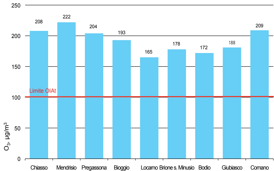
Figura 13: 98° percentile mensile massimo nel 2010
