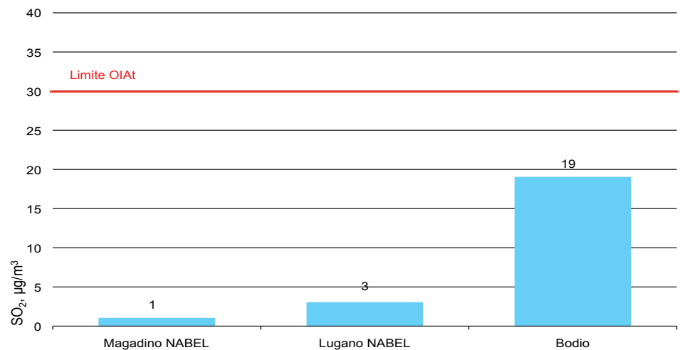
Figura 16: Medie annue di diossido di zolfo in Ticino, 2010
