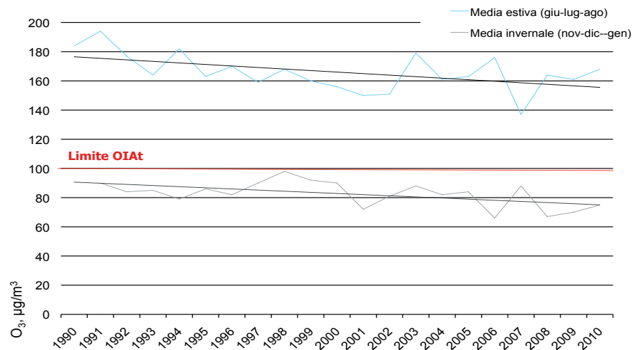
Figura 15: Evoluzione del 98° percentile mensile per l'ozono a Brione sopra Minusio, 1990 – 2010
