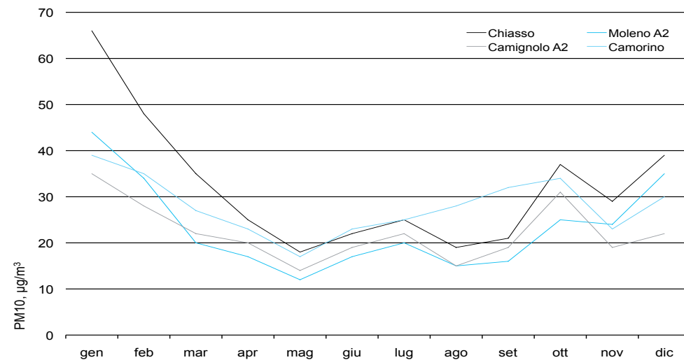
Figura 23: Andamento delle medie mensili delle polveri sottili, PM10, in Ticino, 2010
