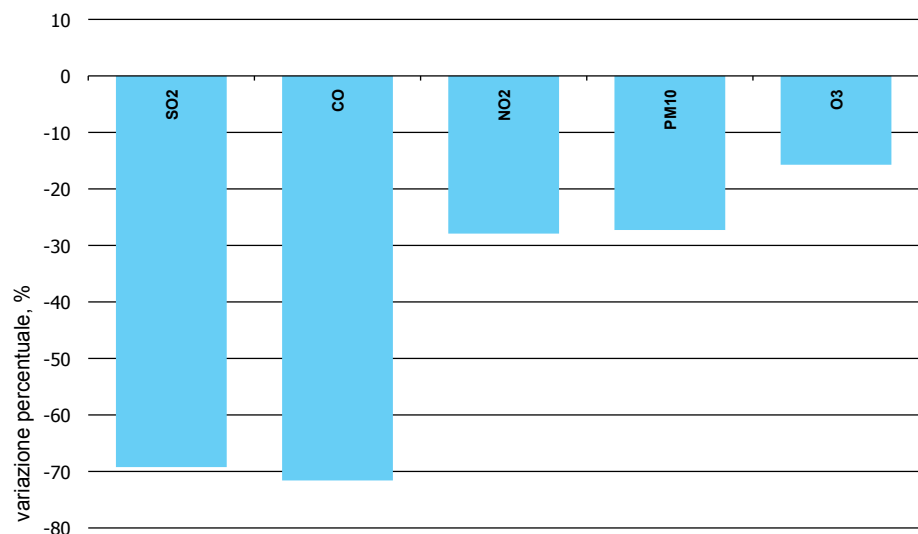
Figura 4: Evoluzione dell'inquinamento atmosferico tra il 1990 e il 2010 per le principali sostanze inquinanti
