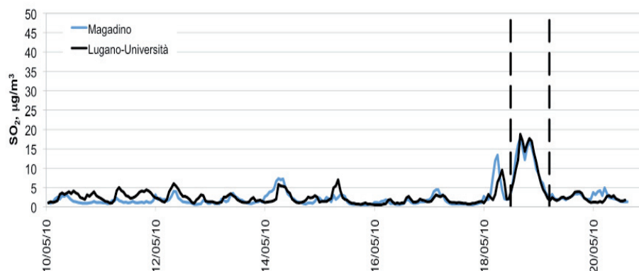
Figura 31: Andamento del diossido di zolfo, SO 2 , dal 10.05.2010 al 20.05.2010
