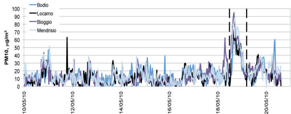
Figura 29: Andamento delle PM10 in Ticino dal 10.05.2010 al 20.05.2010
