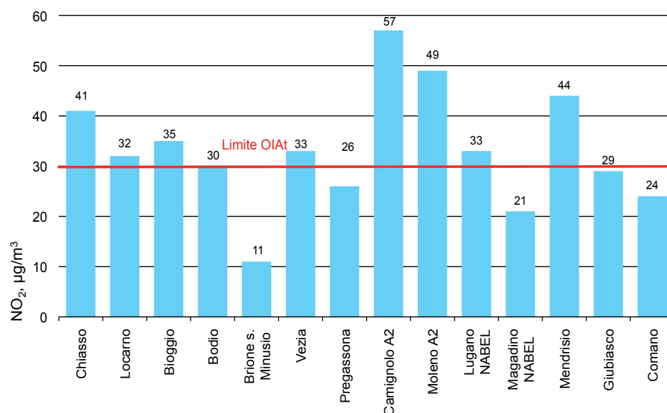
Figura 9: Medie annue di diossido di azoto in Ticino nel 2010
