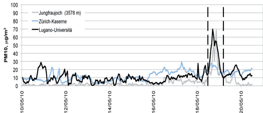
Figura 30: Andamento delle PM10 in Svizzera dal 10.05.2010 al 20.05.2010
