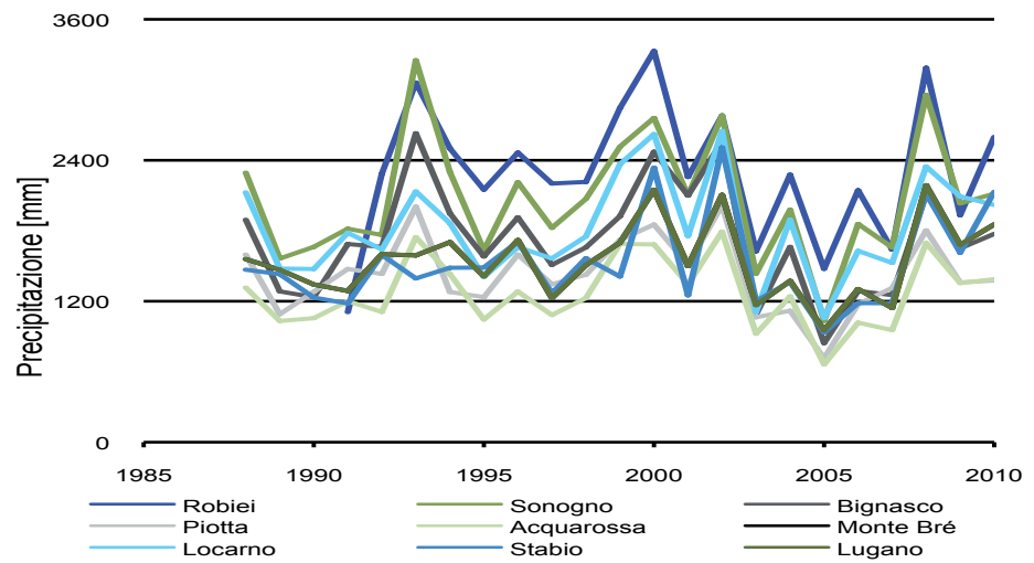
Figura 27: Precipitazione annua; dati MeteoSvizzera
