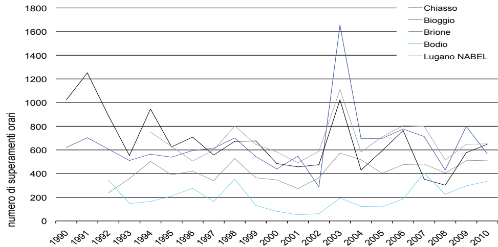
Figura 14: Evoluzione del numero di superamenti del limite orario per l'ozono, 1990 – 2010
