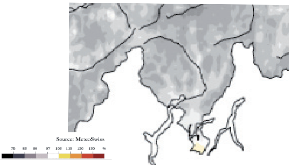
Figura 6b: Deviazione dalla norma dell'irraggiamento in Ticino per il 2010
