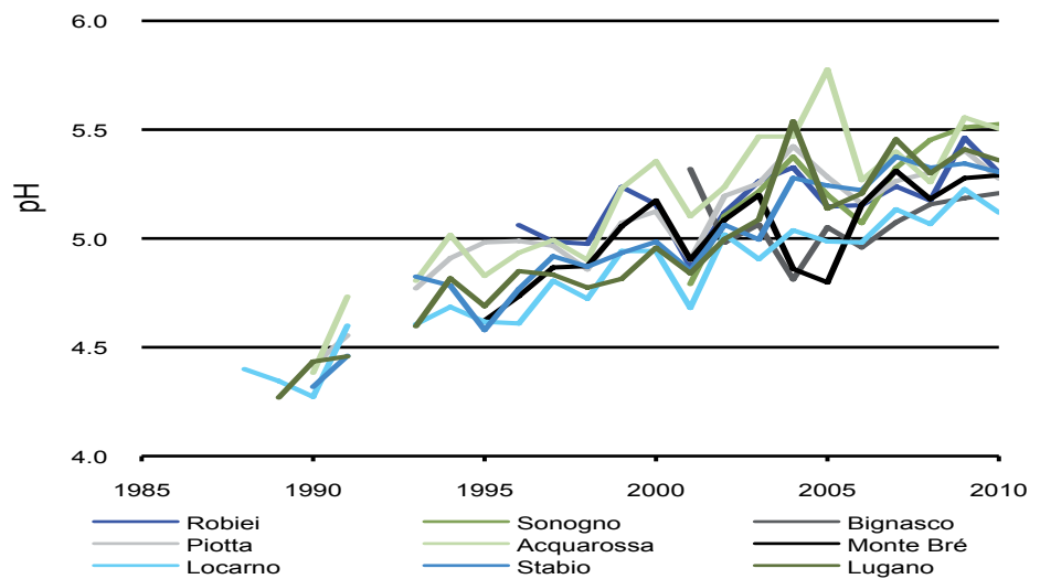
Figura 28: Variazione temporale del pH medio annuo
