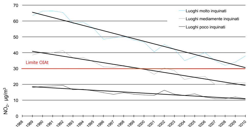
Figura 11: Evoluzione delle medie annue di diossido di azoto in località, poco, mediamente e molto inquinate tramite campionatori passivi, 1989 - 2010
