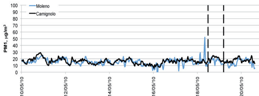
Figura 32: Andamento delle polveri ultrafini, PM1, dal 10.05.2010 al 20.05.2010
