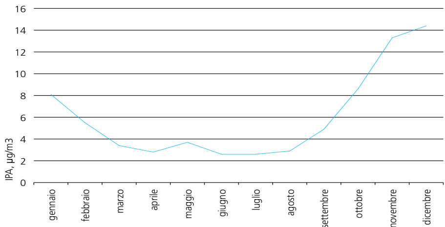
Figura 21: Andamento delle medie mensili degli idrocarburi policiclici aromatici a Comano, 2010
