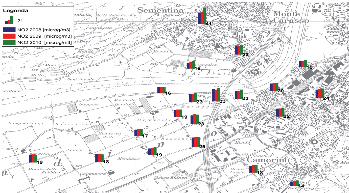
Figura 35: Concentrazioni medie annue di diossido di azoto per il 2008 (blu), 2009 (rosso) e 2010 (verde) nei dintorni dell'impianto cantonale di termovalorizzazione dei rifiuti. Il valore numerico indica la concentrazione in \mu\text{g}/\text{m}^3 nel 2010 (valore limite OIAI per il diossido di azoto: 30 \mu\text{g}/\text{m}^3 ).
