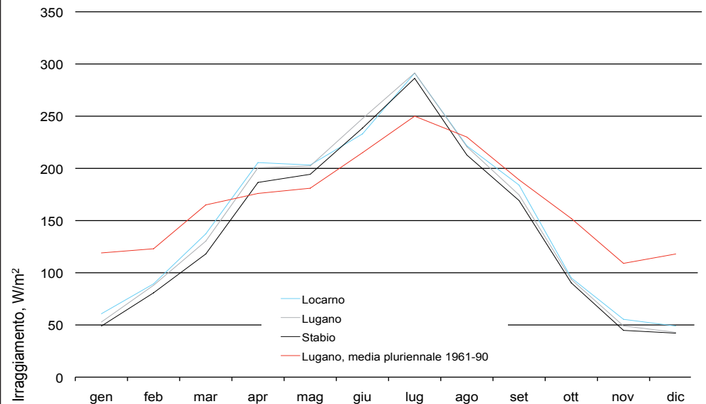
Figura 5b: Irraggiamento, medie mensili
