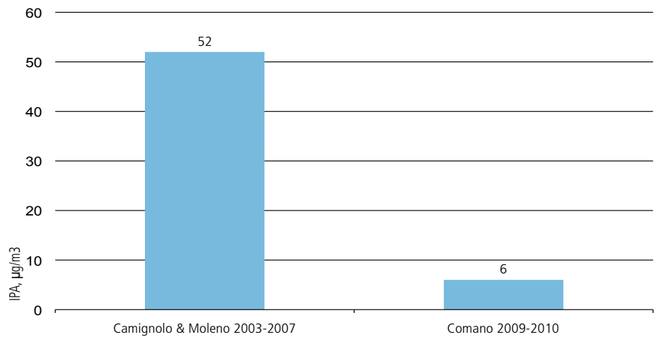
Figura 20: Confronto fra le medie annue degli idrocarburi policiclici aromatici a Camignolo e Moleno (2003-2007) e Comano (2009-2010)
