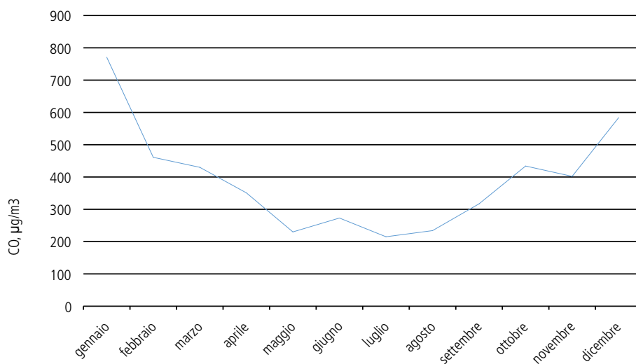
Figura 18: Medie mensili del monossido di carbonio a Lugano NABEL, 2010
