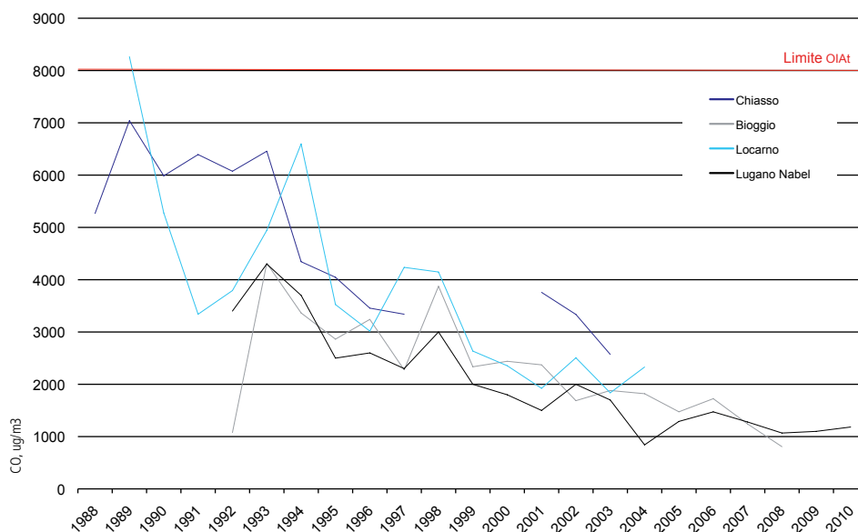
Figura 19: Evoluzione della media giornaliera massima di monossido di carbonio in Ticino 1988-2010
