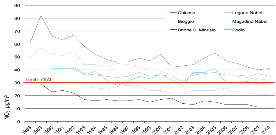
Figura 10: Evoluzione delle medie annue di diossido di azoto in Ticino, 1988 – 2010
