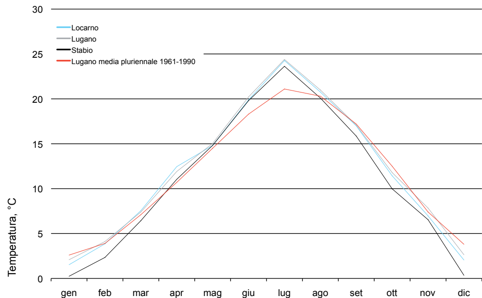
Figura 5a: Temperature, medie mensili
