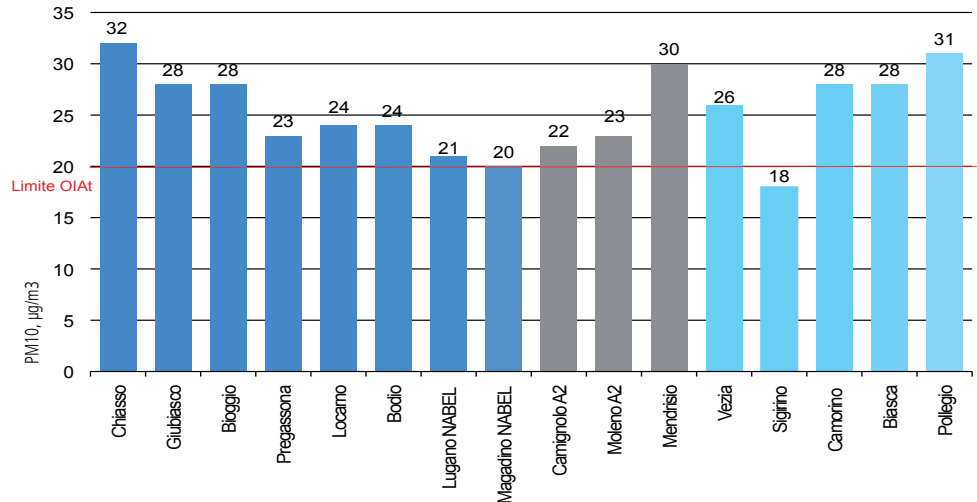
Figura 22: Medie annue delle polveri sottili, PM10, in Ticino, 2010
